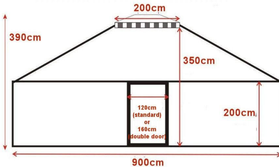
Yurt 9m afmetingen
