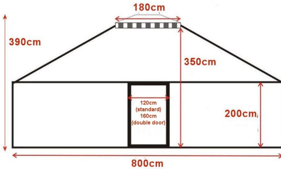
Yurt 8m afmetingen
