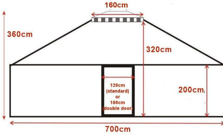
Yurt 7m afmetingen
